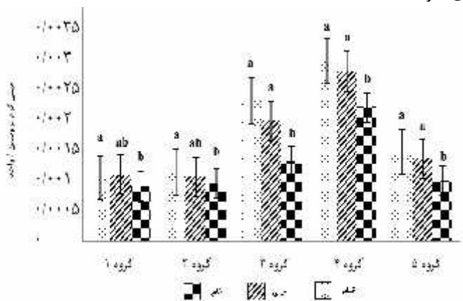
شکل ۲: تغییرات فعالیت آنزیم تریپسین در بخش‌های مختلف روده ماهی سفیدک سیستان (گروه‌های ۱ تا ۴ از ماهیان وحشی و گروه ۵ از ماهیان پرورشی می‌باشد) ( p > 0.05 )
