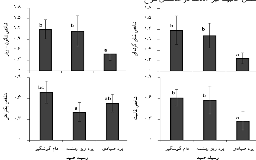
شکل 5: میانگین ( \pm انحراف معیار) شاخص‌ها در روش‌های مختلف صید ماهیان در منطقه جنوب شرقی دریای خزر (گهرباران) حروف مشابه کوچک لاتین گروه‌های همسان در سطح 5 درصد خطا را نشان می‌دهد.
