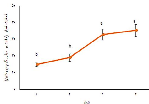
شکل ۲: نمودار میانگین و خطای معیار میزان فعالیت آنزیم لیپاز روده ماهی کفال خاکستری در تیمارهای مختلف (۰، ۱۵، ۵۰، ۱۰۰ گرم عصاره جلبک جانی در هر کیلوگرم غذا) در پایان دوره آزمایش حروف نامشابه در هر ستون نشان دهنده اختلاف معنی دار بین تیمارها است ( p < 0.05 ).
