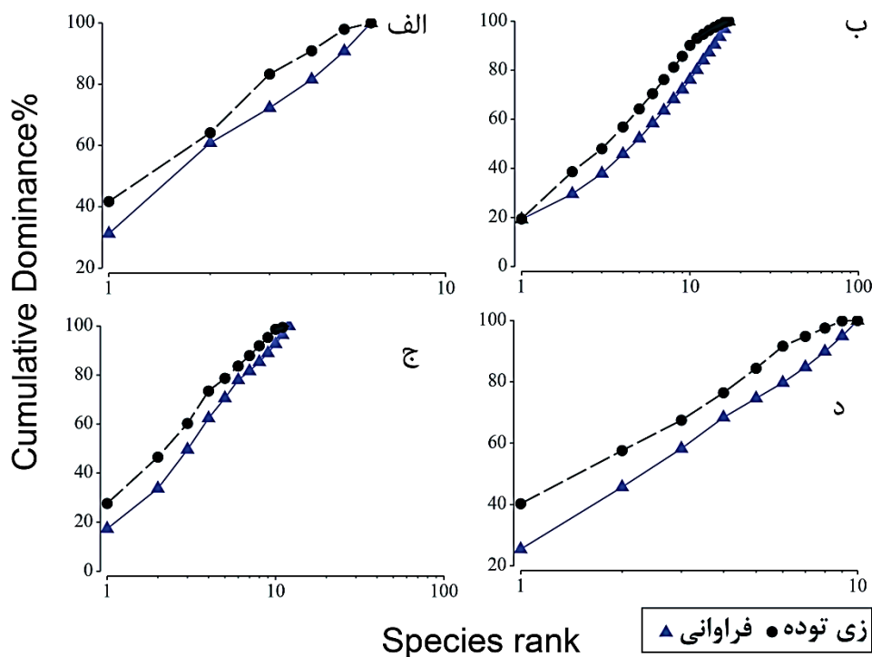
شکل ۳: نمودارهای منحنی‌های ABC در مناطق دارای پوشش گیاهی (Vegetated) بندرخمیر و طبل. "الف" و "ب": طبل، به ترتیب ترانسکت ۱ و ۲. "ج" و "د": بندرخمیر، به ترتیب ترانسکت ۳ و ۴
