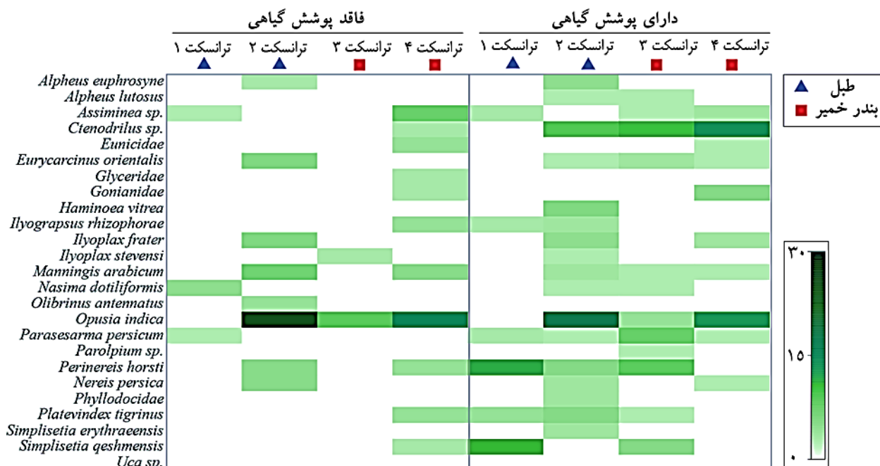
شکل ۲: گونه‌های شناسایی شده به همراه فراوانی آن‌ها (تعداد در مترمربع) در دو منطقه طبل و بندرخمیر در نواحی دارای پوشش گیاهی حرا (شامل ریشه درختان حرا) و فاقد پوشش گیاهی (بسترهای گلی اطراف نهرهای جنگل‌های حرا)، از داده‌های فراوانی، ریشه دوم گرفته شده است.
