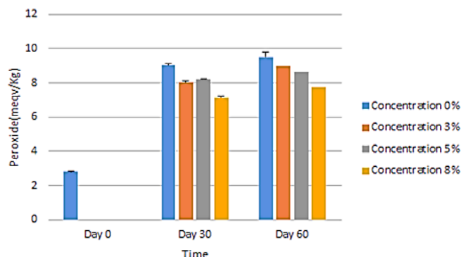
شکل ۴: نمودار تغییرات شاخص پراکسید (Peroxide) در سس مهباه در مدت ۶۰ روز نگهداری در ۴ گروه مورد بررسی
