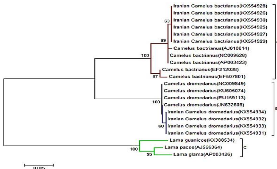
شکل ۳: ترسیم درخت فیلوژنی براساس توالی ژن ۱۶s rRNA میتوکندریایی شترهای ایرانی و سایر توالی‌های این ژن در بانک جهانی ژن به همراه کد دسترسی آن‌ها. اعداد روی گره مربوط به درصد مشابهت درون گروهی حاصل از ۱۰۰۰ مرتبه نمونه‌گیری می‌باشد.
