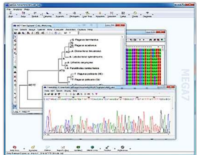
شکل ۴: آنالیز فیلوژنتیکی با استفاده از نرم افزار MEGA
