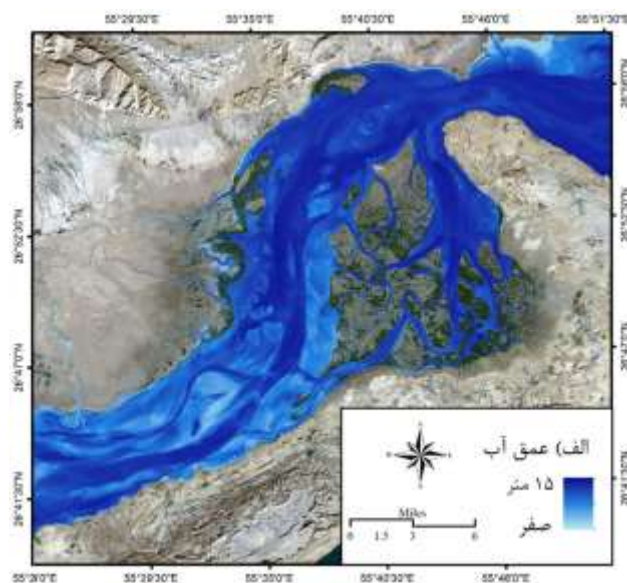
شکل ۳: نقشه عمق آب تهیه شده از پردازش تصاویر ماهواره Landsat 8-OLI
