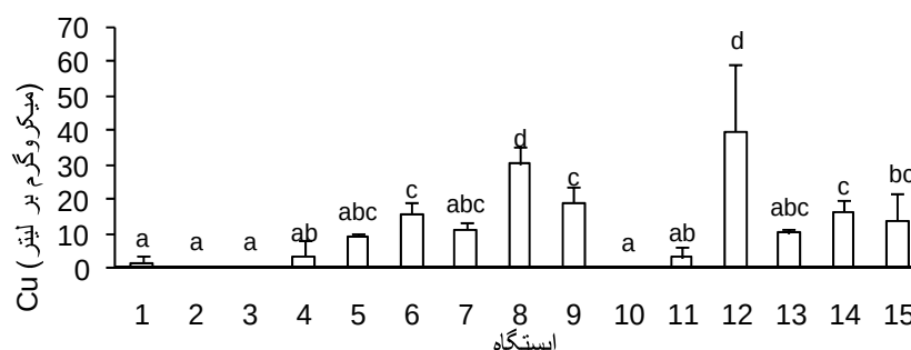
نمودار ۱: میزان مس (میانگین و انحراف معیار) در رودخانه گرگانود در ایستگاههای مختلف (بهار ۱۳۸۸) حروف لاتین غیریکسان نشانگر وجود اختلاف معنی‌دار می‌باشند ( P<0.05 ).
