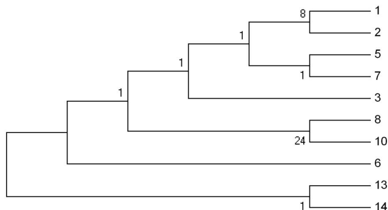
شکل ۲: درخت فیلوژنتیک به روش پیوند همجواری
