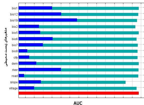
شکل 5: نمودار آزمون جک نایف جهت بررسی میزان نقش هریک از متغیرها در اعتبار مدل
