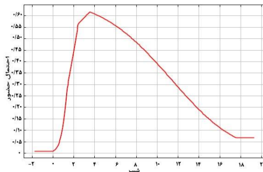
شکل 7: منحنی پاسخ شیب
