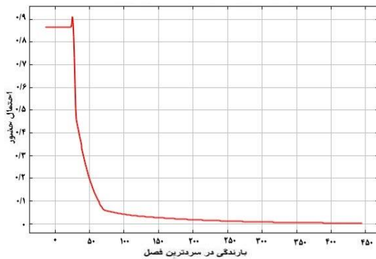
شکل 6: منحنی پاسخ بارندگی در سردترین فصل
