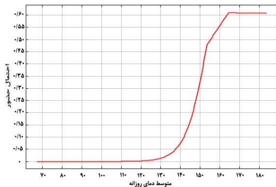
شکل 8: منحنی پاسخ متوسط دمای روزانه
