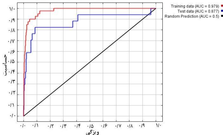
شکل 2: منحنی ROC جهت بررسی اعتبار مدل
